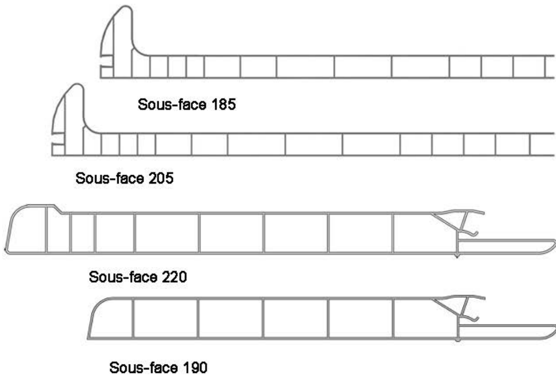
Figure 1.3 : Profil d'habillage du rail aluminium
