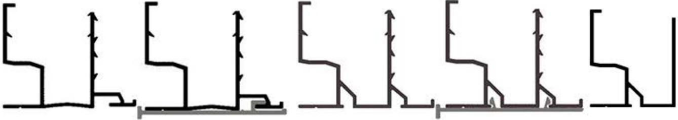
Figure 1.1 : Rails aluminium extérieurs sans et avec le cache rail
